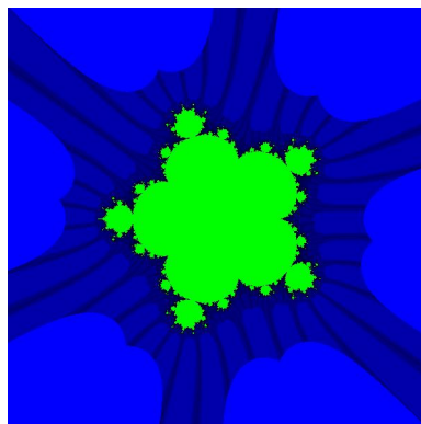
(d) z^6 + c ( d = 6 )
